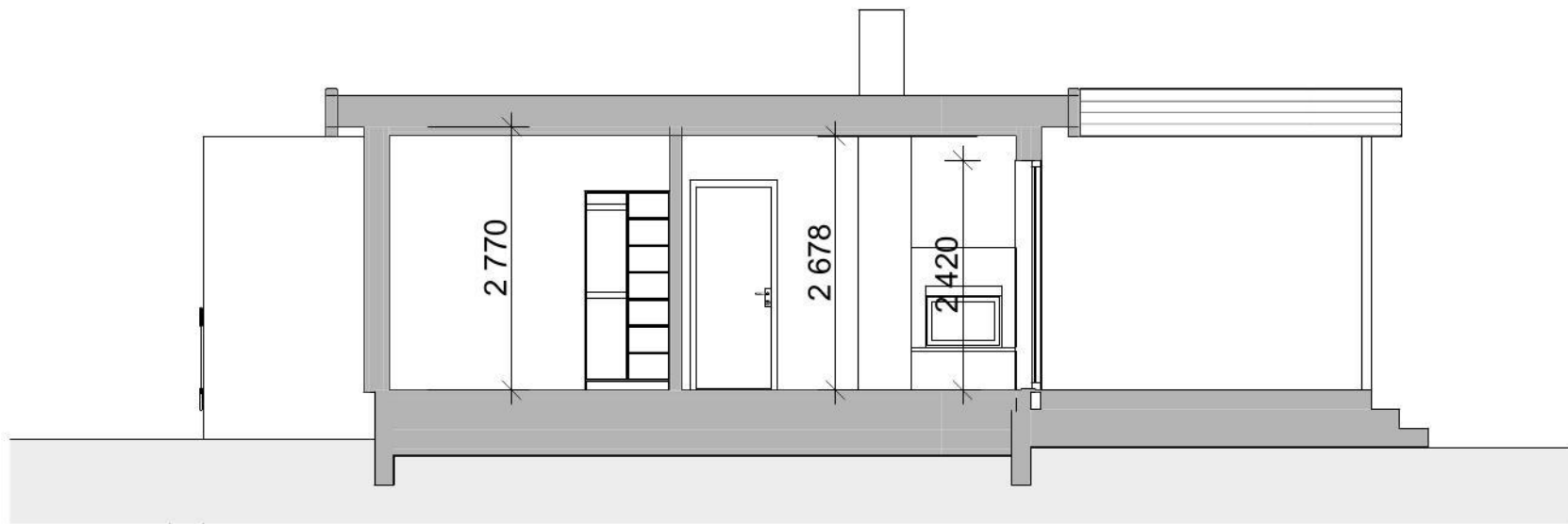
1:100 Snitt A
